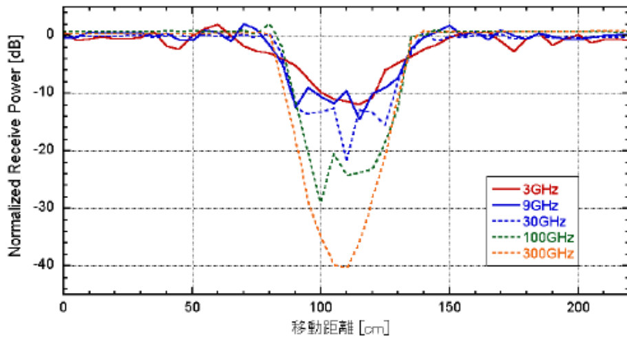
(Fig. 3-2 遮蔽ロスの測定結果例 [1])
