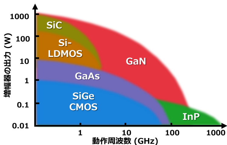
Fig. 4-8 周波数と増幅器出力の関係
