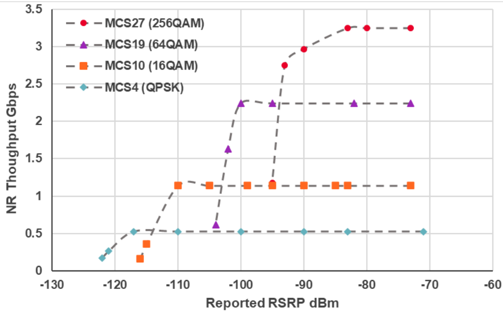
Fig. 5-2 5Gミリ波の端末受信スループット
