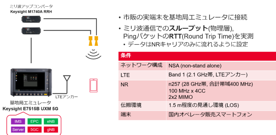
Fig. 5-1 市販ミリ波端末の性能評価例 (Keysight提供)
