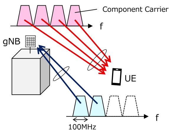
Fig. 4-10 ミリ波キャリアアグリゲーション (CA)
