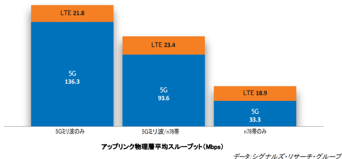
Fig. 5-7 屋外における5Gミリ波上りリンクスループット移動測定
