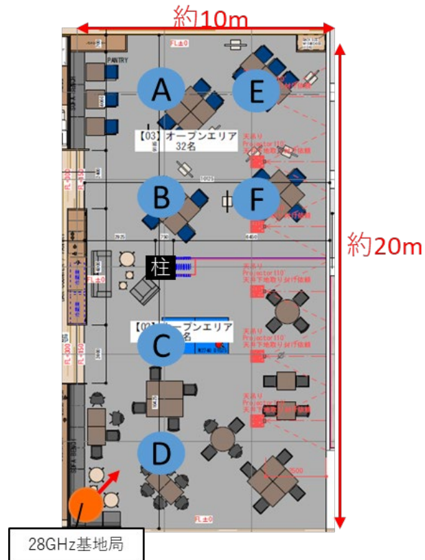
Fig. 5-4 5Gミリ波スループットの屋内測定
