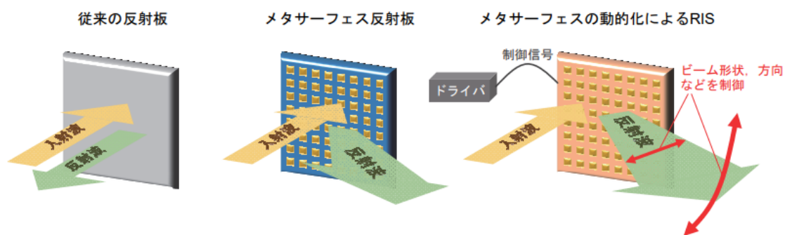
Fig. 4-7 メタサーフェス技術を用いたRISの概念図
