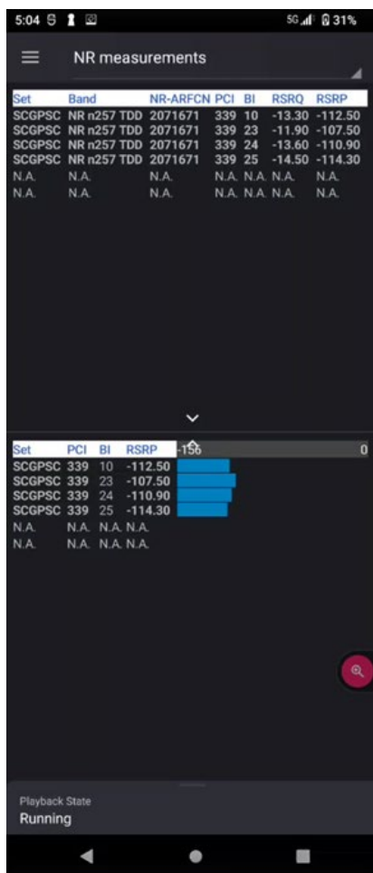
Fig. 9-8 Nemo Handy 市販スマホ上でFR2モニタ例 (Keysight提供)
