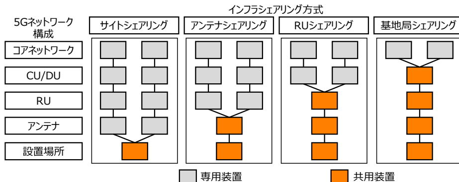
Fig. 4-9 インフラシェアリング方式の比較
