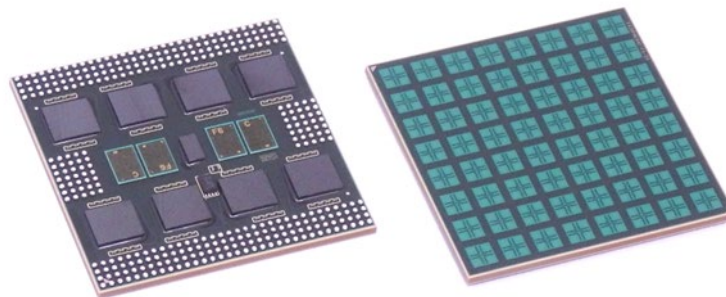
Fig. 9-7 基地局向け8x8アレイアンテナモジュール(24 – 29 GHz) (フジクラ製)
