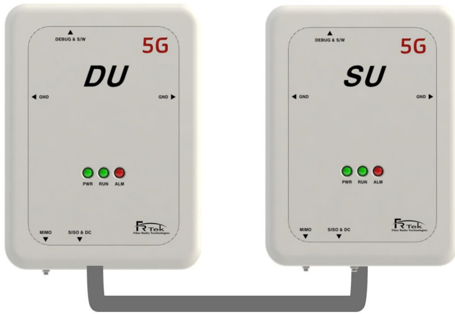
Fig. 9-11 ドナーユニットとサービスユニットの2つの筐体で構成されるミリ波レピータ (FR-Tech製)
