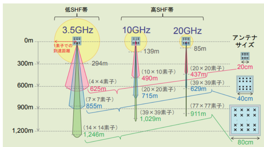
Fig. 4-2 ビームフォーミングの効果
