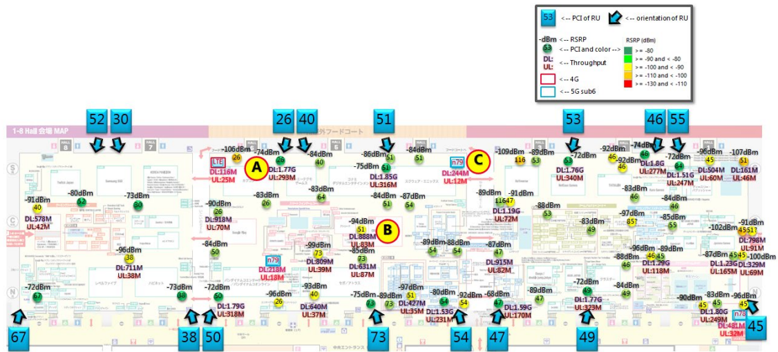
Fig. 5-11 ゲームイベント会場内での測定
