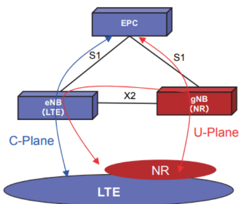
Fig. 4-11 LTE-NR Dual Connectivity接続イメージ
