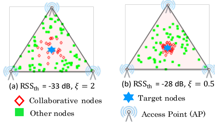
Fig. II-1.5-1 Simulation setup [8].
